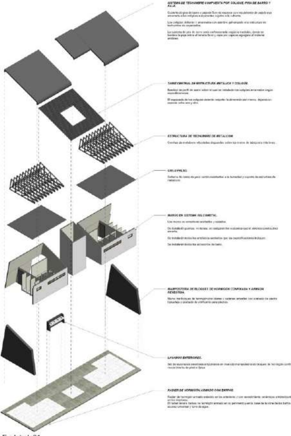
2 Explotada01
