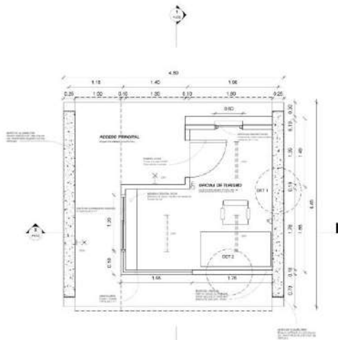
1 Nivel 1 1:25
