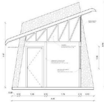
2 Sección 1 1:25
