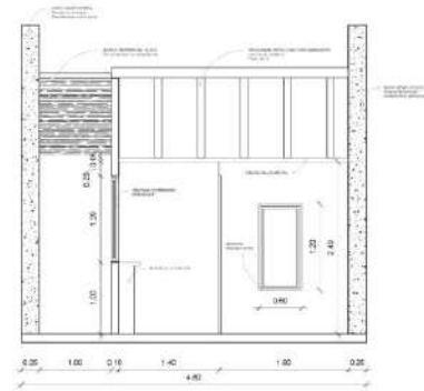
6 Sección 2 1:25
